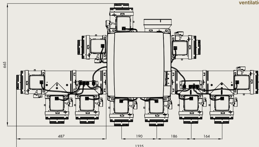
Un seul conduit aéraulique
