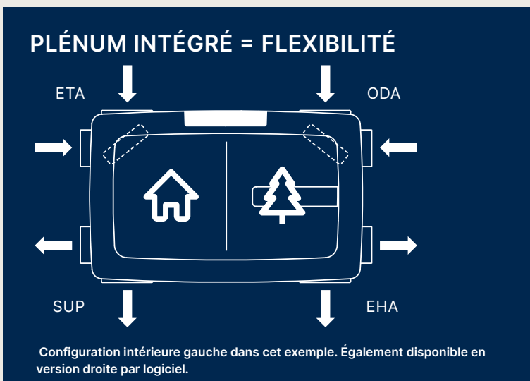
INSTALLATION HORIZONTALE SUR LE MUR Espace bas et large
