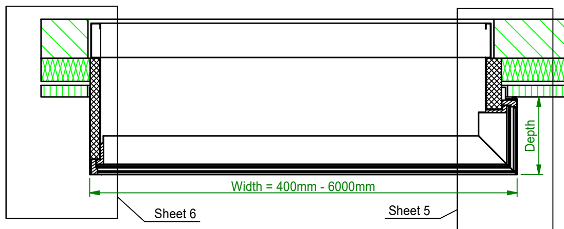
Section B-B ( 1 : 20 )
