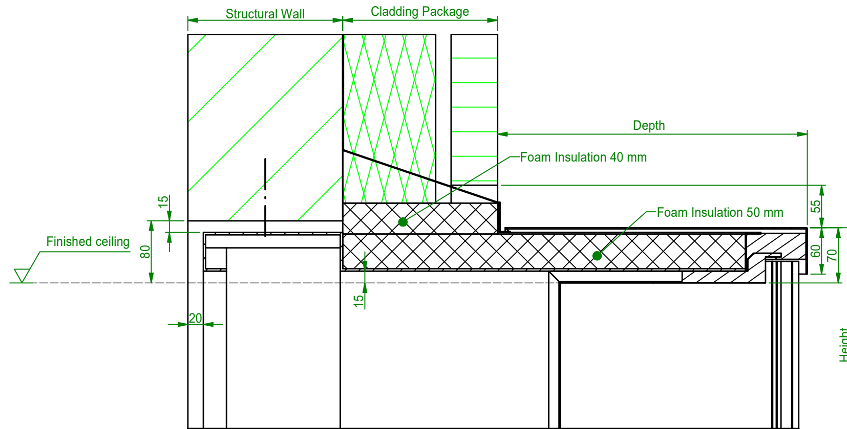
Sheet 3 ( 1 : 5 )
