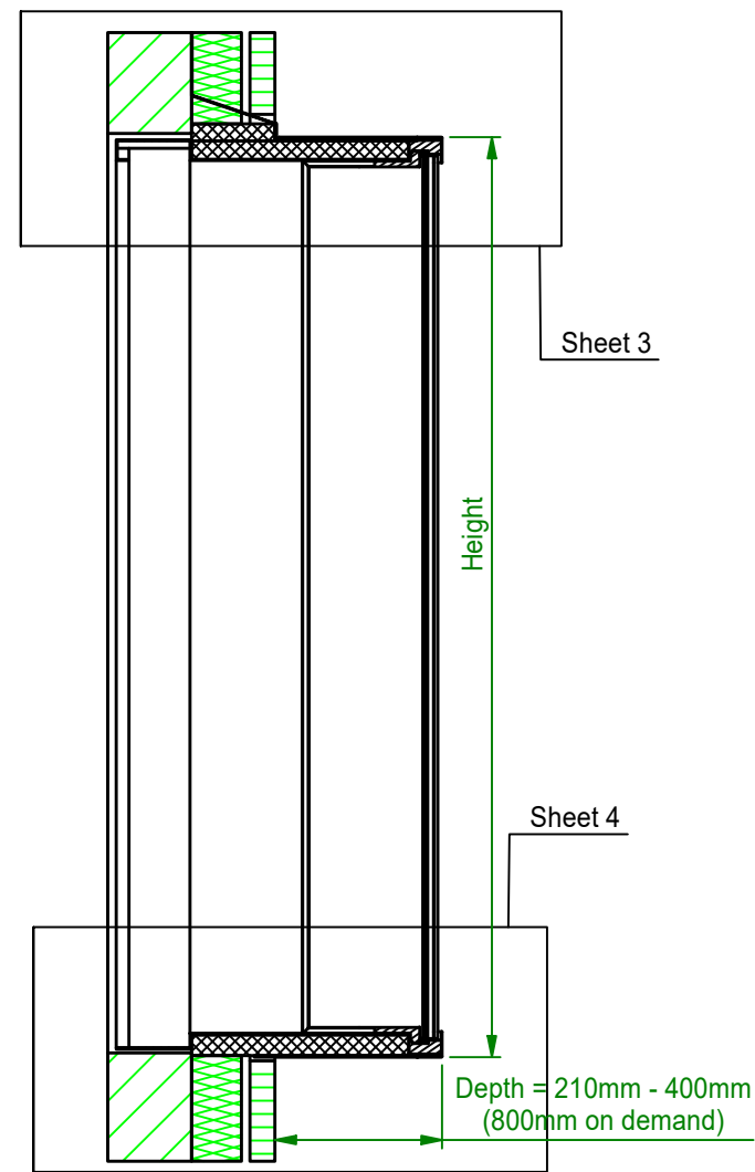
Section A-A ( 1 : 20 )
